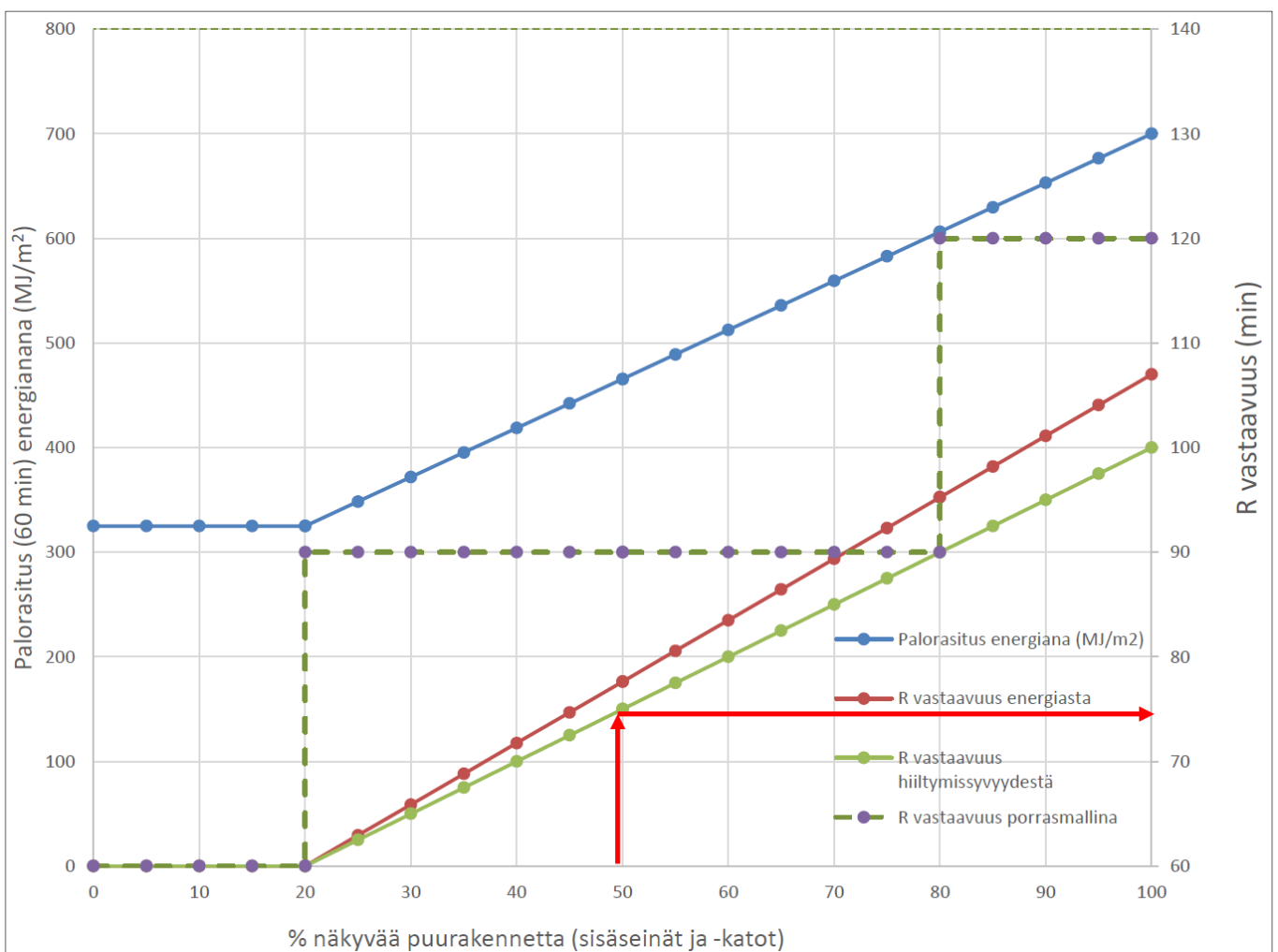
Kuva 1. Näkyvän puupinnan vaikutus palo-osaston rakennusosien luokkavaatimukseen (lähde: Puutuoteteollisuus ry).
